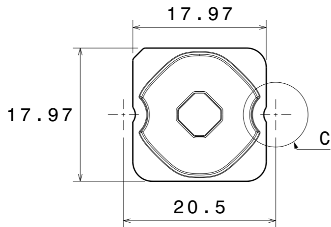
Top view Scale: 2:1
