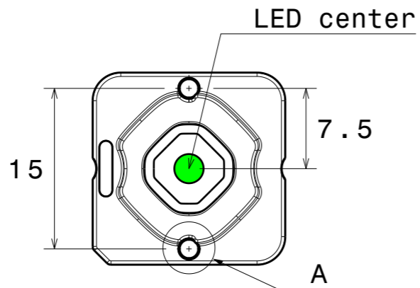
Bottom view Scale: 2:1
